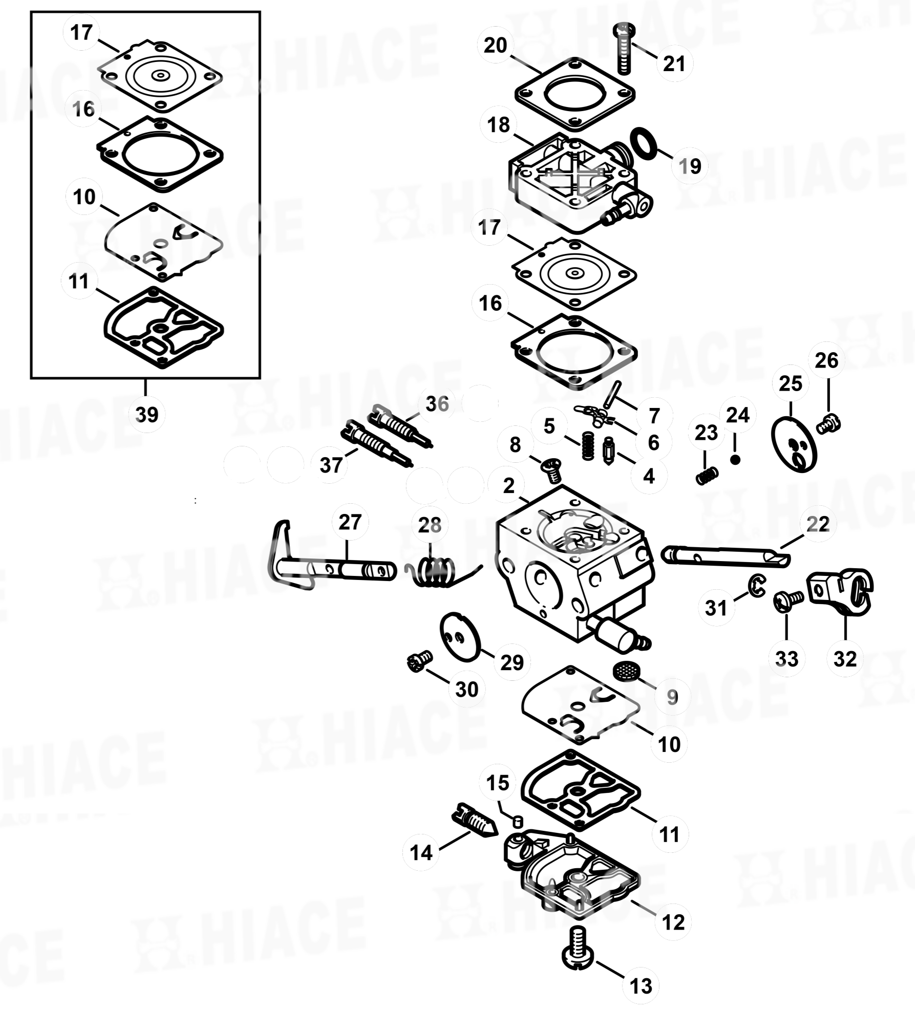
化油器 Carburetor 413/21、4134/22、4134/23
