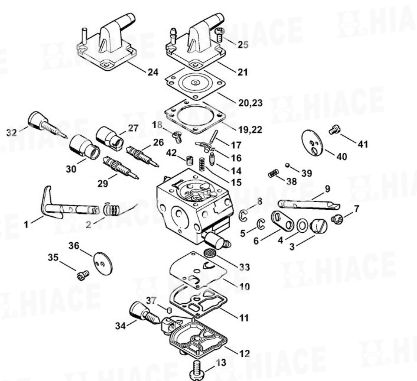
化油器 Carburetor C1Q-S161、-S162、-S163、-S164、 -S82、-S83、-S138、-S139
