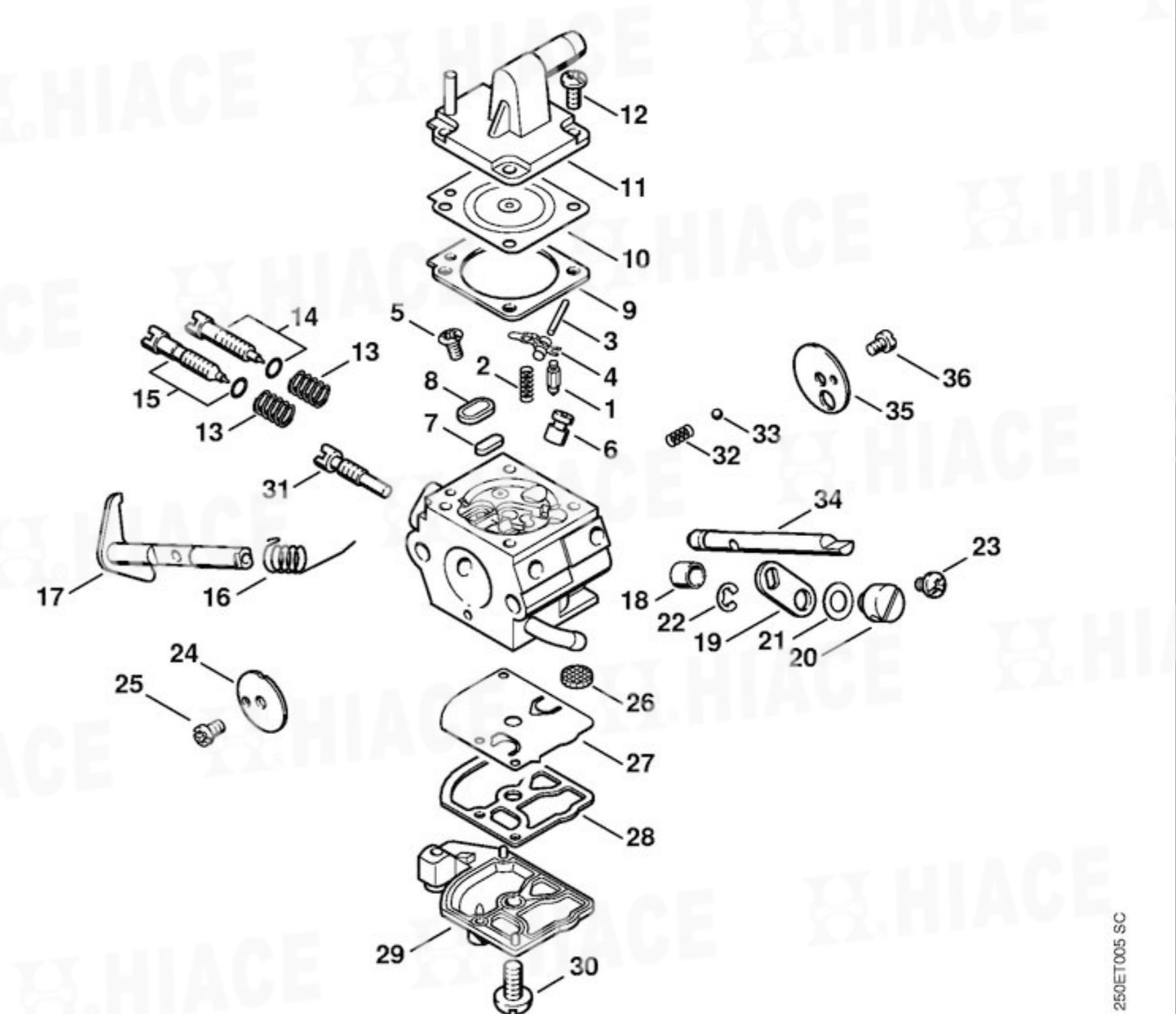
化油器 Carburetor C1Q-S35(19.98)
