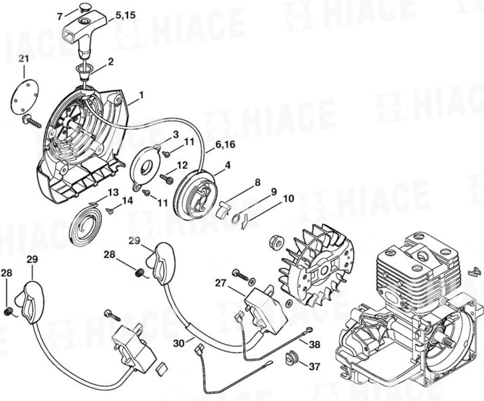
啟動裝置、點火系統 Rewind starter, Ignition system 809 249 646
