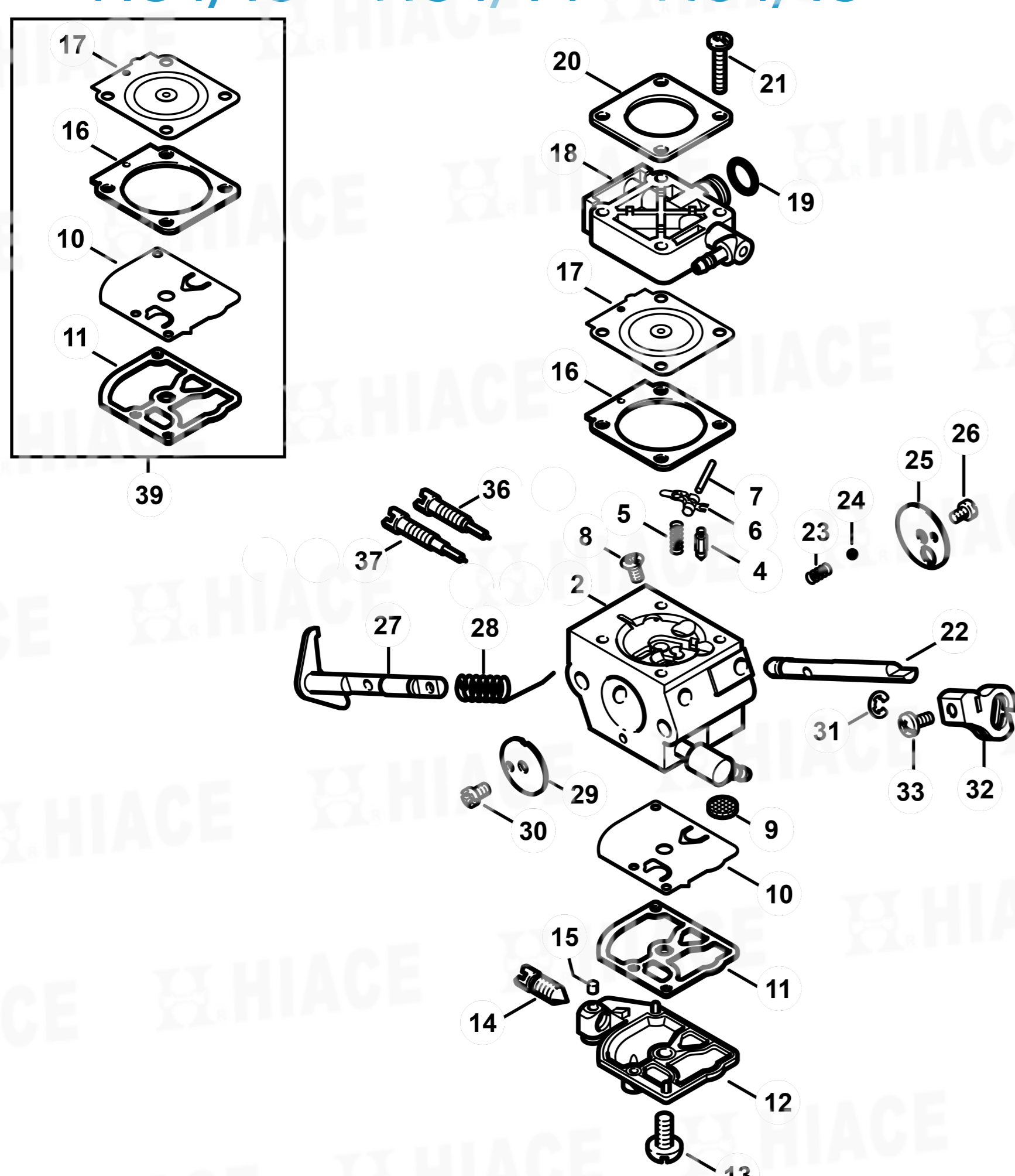
化油器 Carburetor 4134/13、4134/14、4134/15
